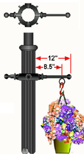
WF10-PVL12-01M0-A490
